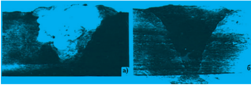
Рис. 5 Макроструктура сварных соединений стали 09Г2СЦТР (оптимального состава): а - ручная сварка; б - автоматическая сварка под флюсом.
