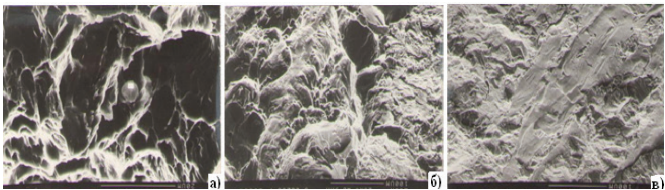
Рис. 4. Микрофрактограммы излома стали 09Г2ГЦТР (x500).
