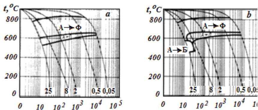
Рис.1. Термокинетические диаграммы превращения переохлажденного аустенита при непрерывном охлаждении стали 09Г2С и 09Г2СЦТР.
