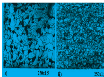
Рис. 2. Микроструктура стали 09Г2С (а) и 09Г2СЦТР (б).
